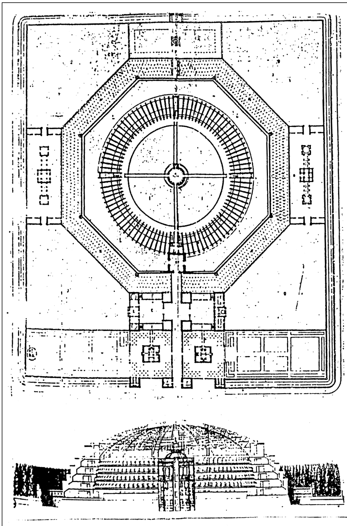
N. Harou-Romain. Projet de pénitencier, 1840.
